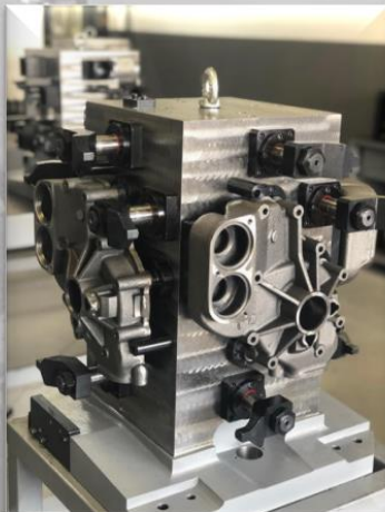
Fixações Hidráulicas para Centros Horizontais
