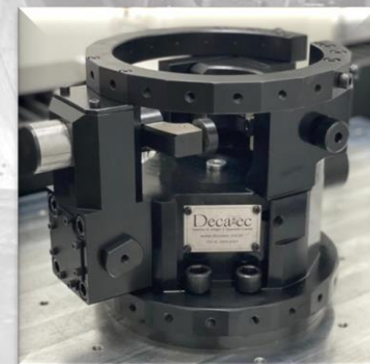
Fixações para tornos cnc
