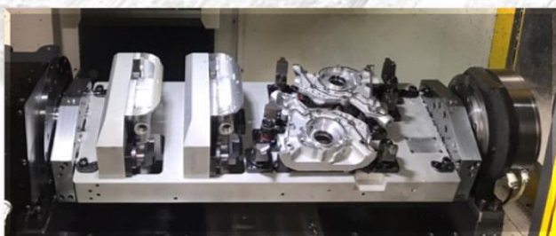
Fixações Hidráulicas para Centros Verticais
